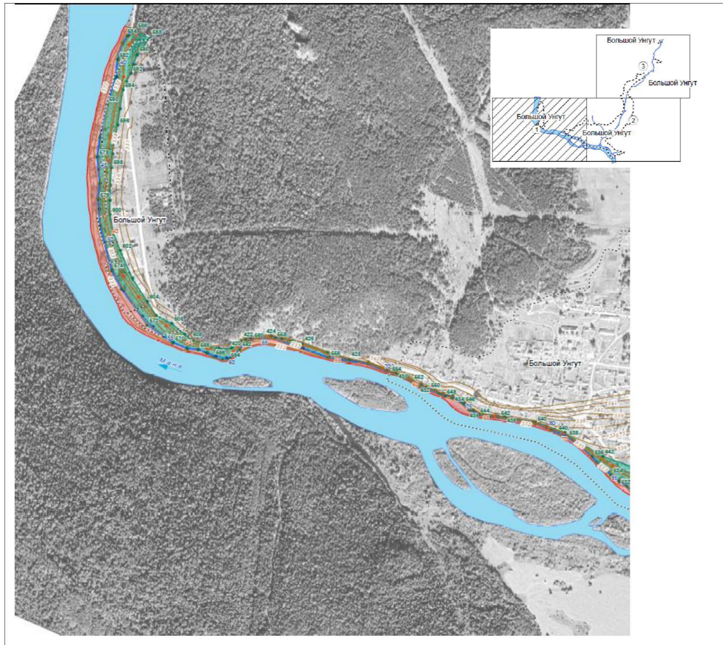
Приложение 6 Карта зон с особыми условиями использования территории п. Большой Унгут, Унгутского сельсовета (зоны затопления, подтопления территорий)
