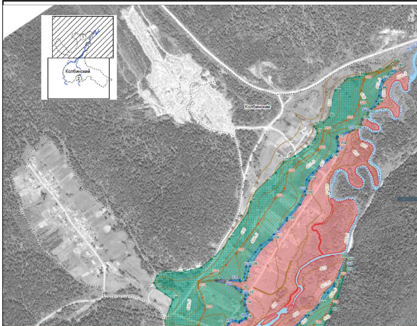
Приложение 5 Карта зон с особыми условиями использования территории п. Колбинский, Колбинского сельсовета (зоны затопления, подтопления территорий)
