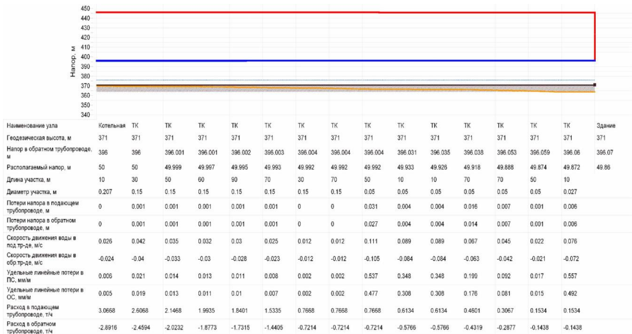
Пьезометрический график №1
