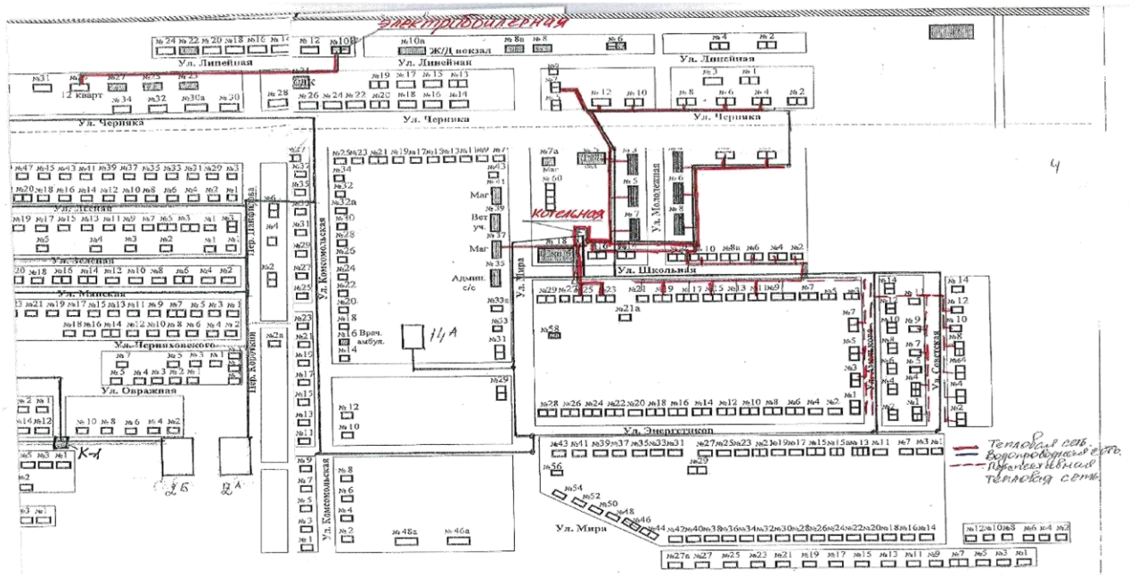
Схема тепловых сетей
